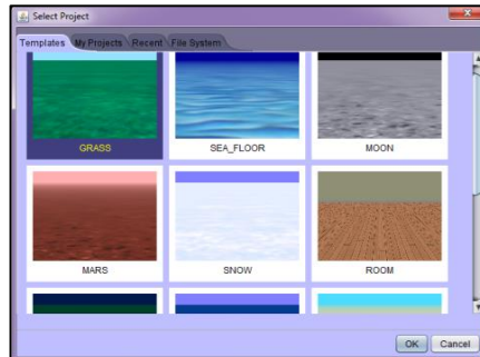
Εικόνα 2 Καρτέλα Templates
